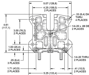
VIEW A-A
