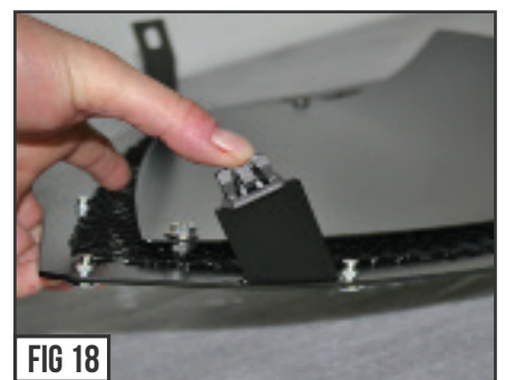
10-32 Flange Nuts
