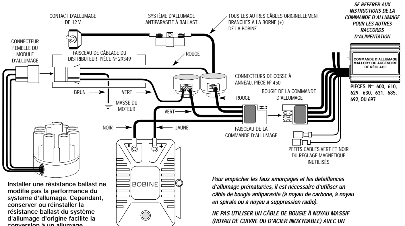
FIGURE 3 SCHÉMA DE CÂBLAGE POUR LES COMMANDES D'ALLUMAGE ÉLECTRONIQUES DE RECHANGE
