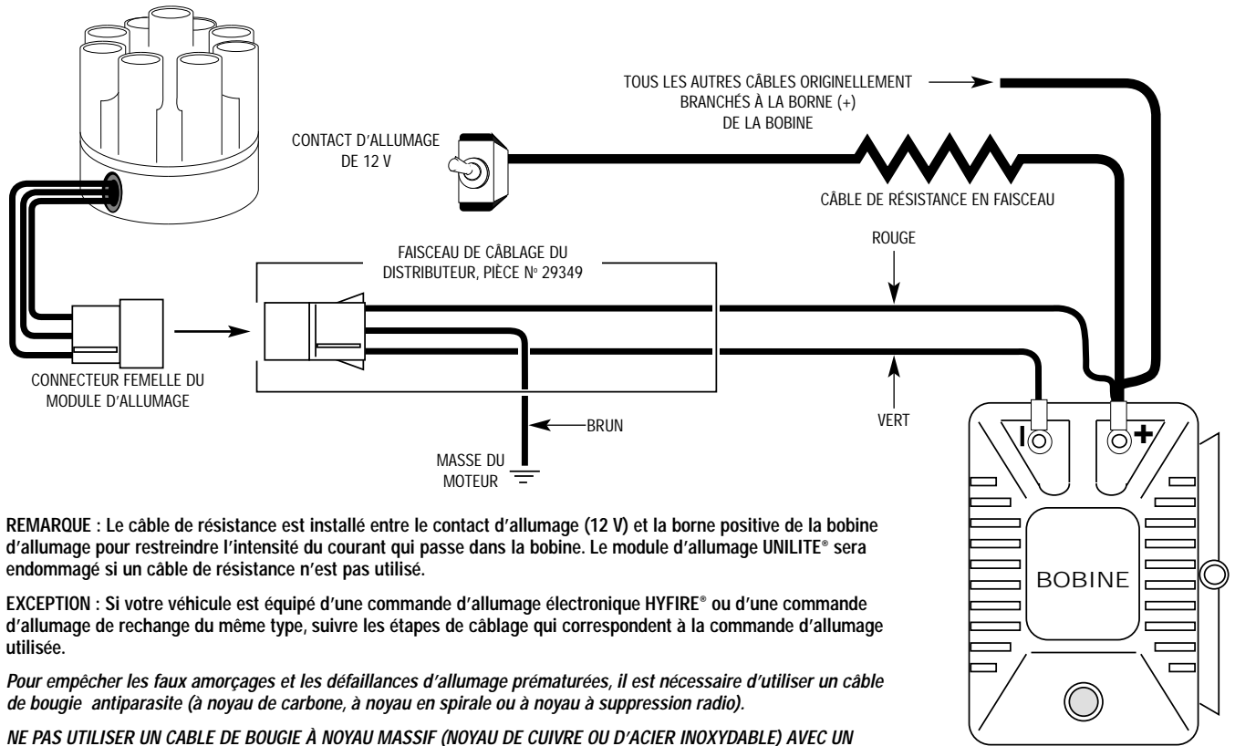
FIGURE 2 SCHÉMA DE CÂBLAGE UNILITE® UTILISANT UN CÂBLE À RÉSTANCE PRIMAIRE DE L'ÉQUIPEMENTIER (OEM)
