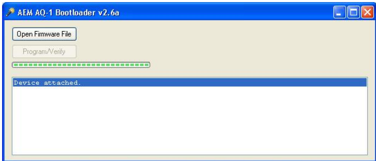
Figure 24. AQ1 Bootloader
