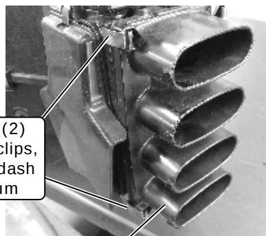
Dash Plenum 625330
